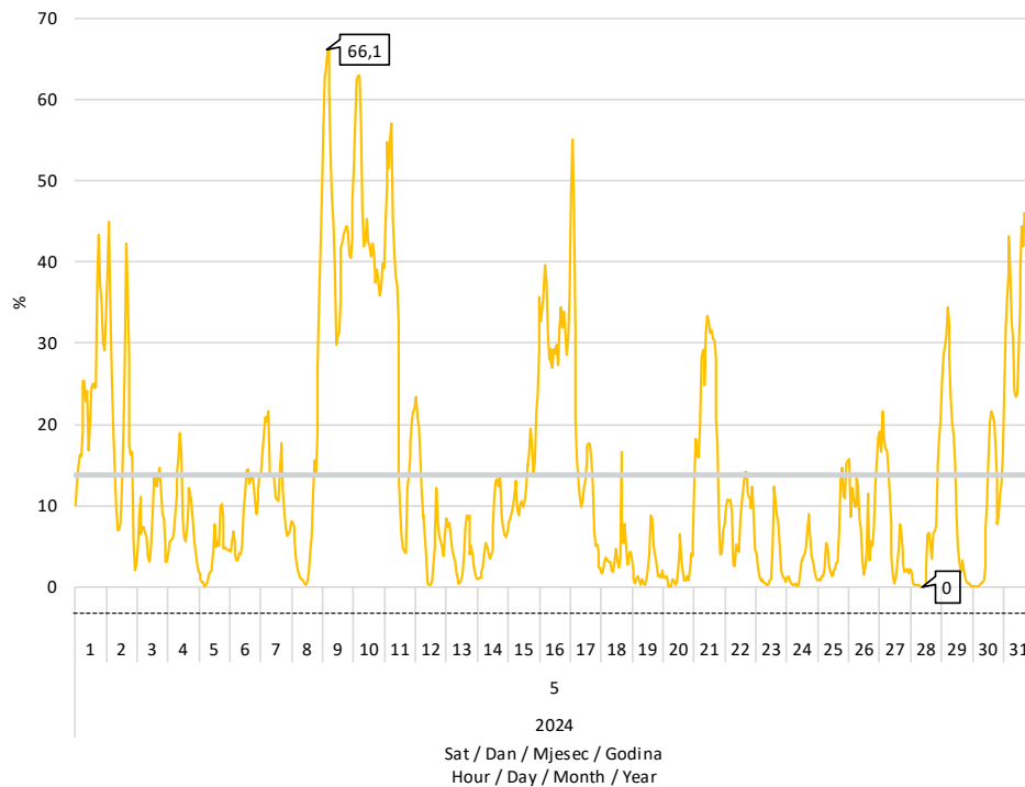
Slika 8 Udio proizvodnje vjetroelektrana u pokrivanju satnog opterećenja elektroenergetskog sustava u svibnju 2024. godine
