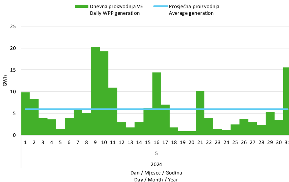
Slika 5 Dnevna proizvodnja svih vjetroelektrana u svibnju 2024. godine Figure 5 Daily generation of all wind power plants in May 2024
