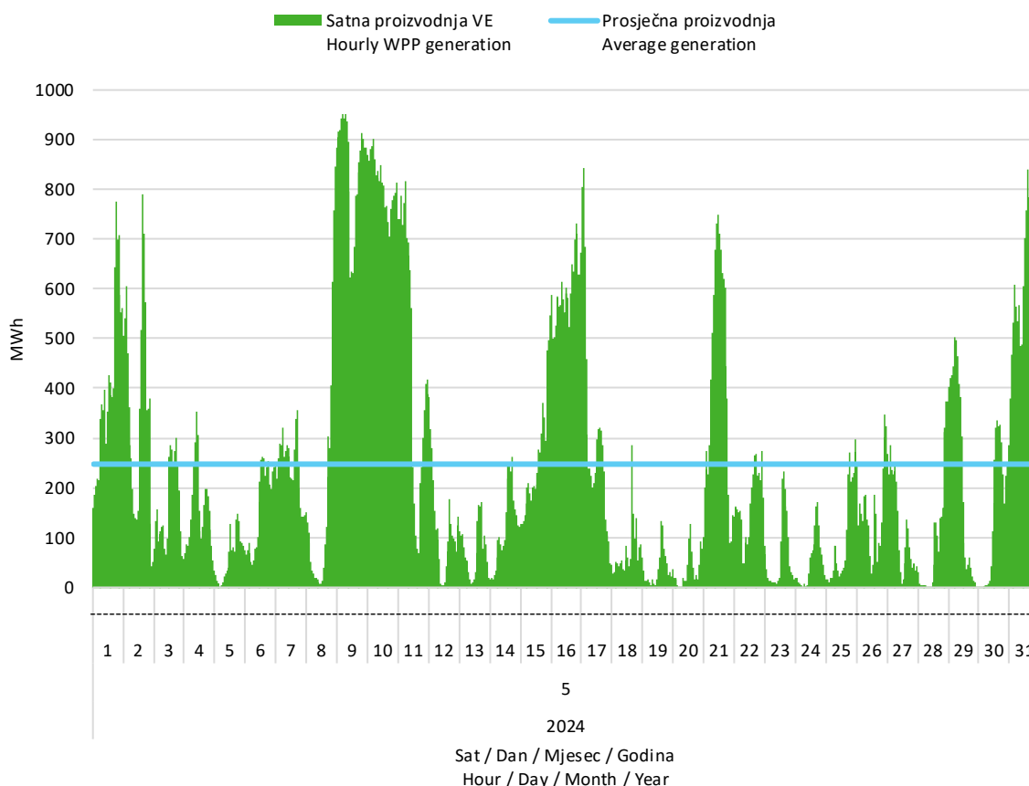
Slika 2 Satna proizvodnja svih vjetroelektrana u svibnju 2024. godine
