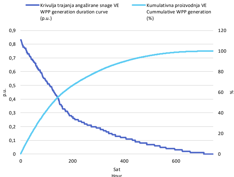
Slika 3 Krivulja trajanja angažirane snage svih VE i kumulativna proizvodnja VE u svibnju 2024. godine u jediničnim vrijednostima
