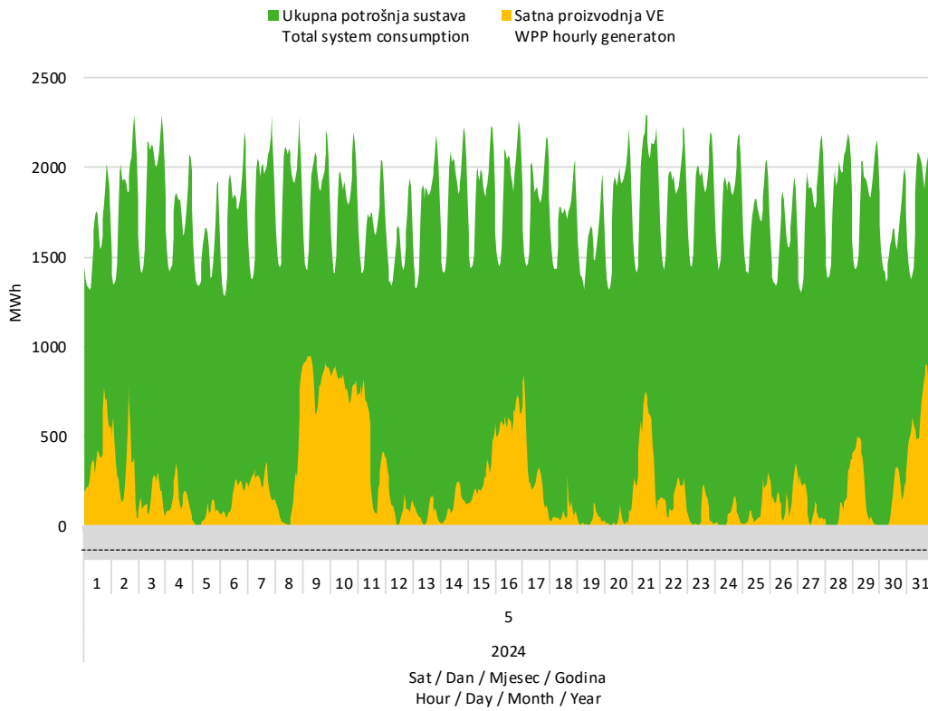
Slika 7 Usporedba satnog dijagrama opterećenja sustava i proizvodnje vjetroelektrana u svibnju 2024. godine
