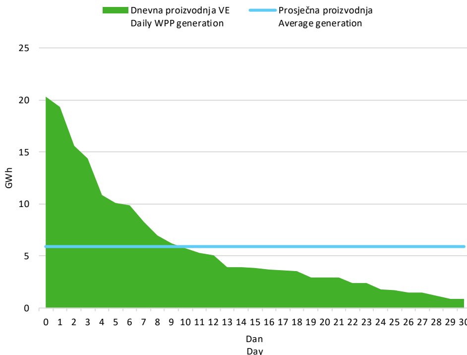
Slika 6 Krivulja trajanja dnevne proizvodnje vjetroelektrana u svibnju 2024. godine
