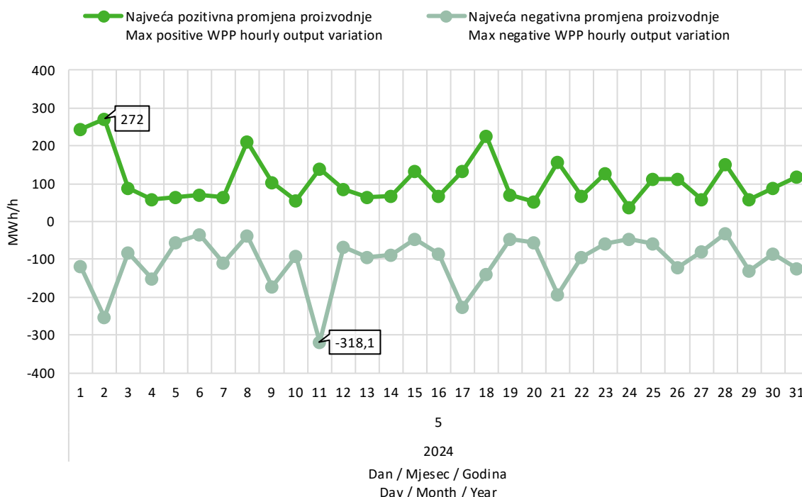
Slika 9 Maksimalna pozitivna i maksimalna negativna promjena satne proizvodnje VE u svibnju 2024. godine
