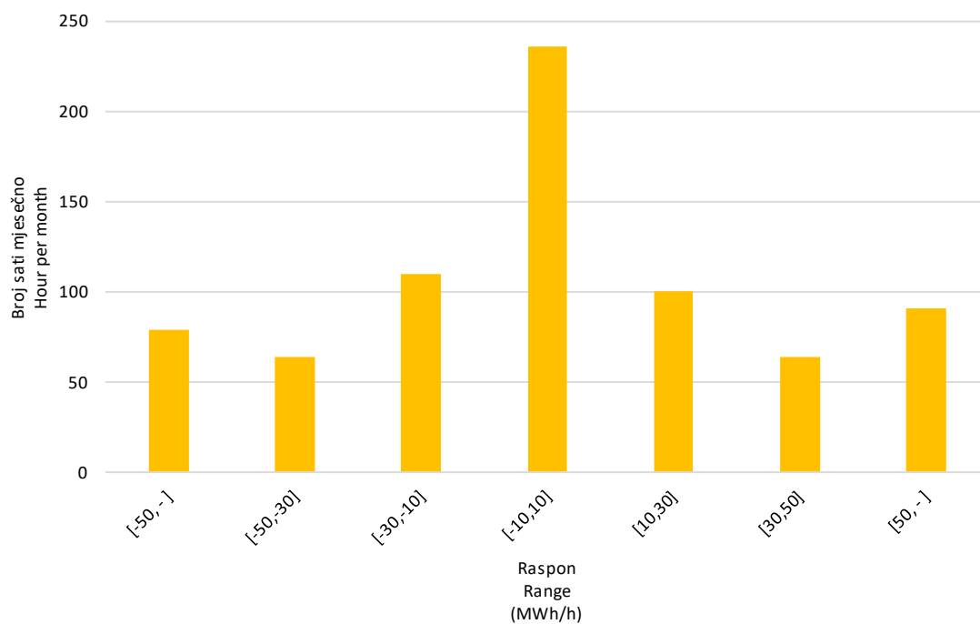
Slika 10 Statistička raspodjela satnih promjena proizvodnje VE u svibnju 2024. godine
